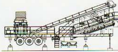
Cono y Criba
