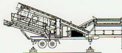
Tolva preclasificadora y Criba
