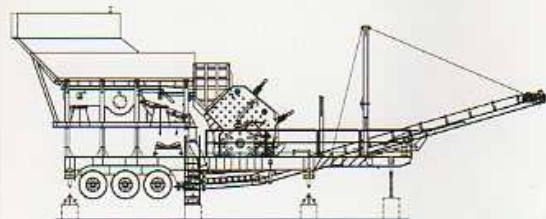
Impactor primario
