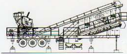
Impactor y Criba
